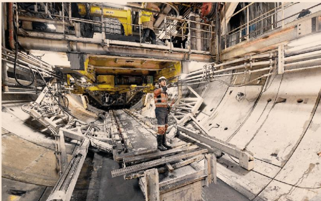
Torino-Lione. I lavori per la realizzazione della linea ad alta velocita
